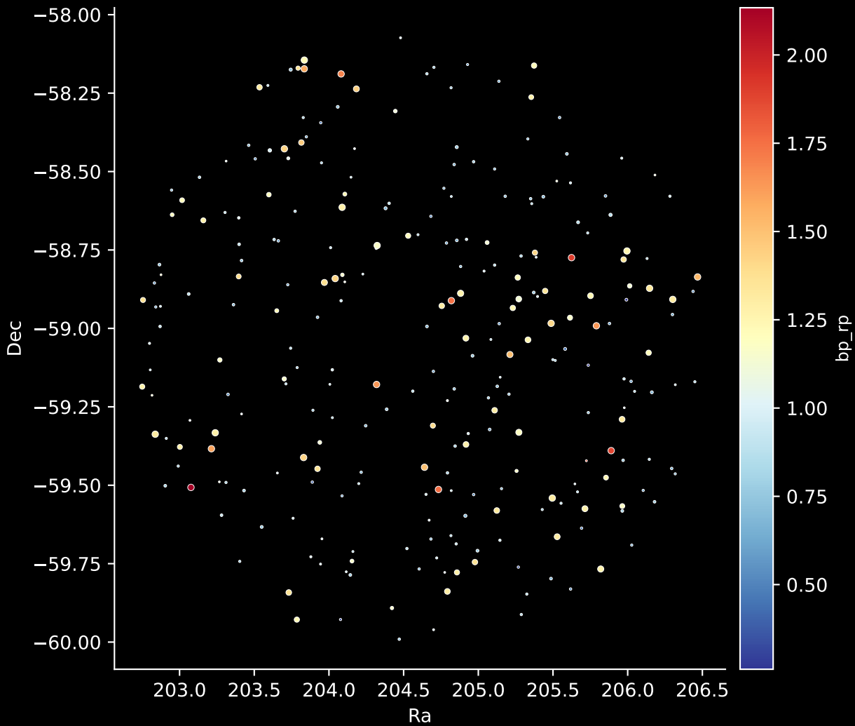
GALAH DR4 Field: [7191] Stars: 270
