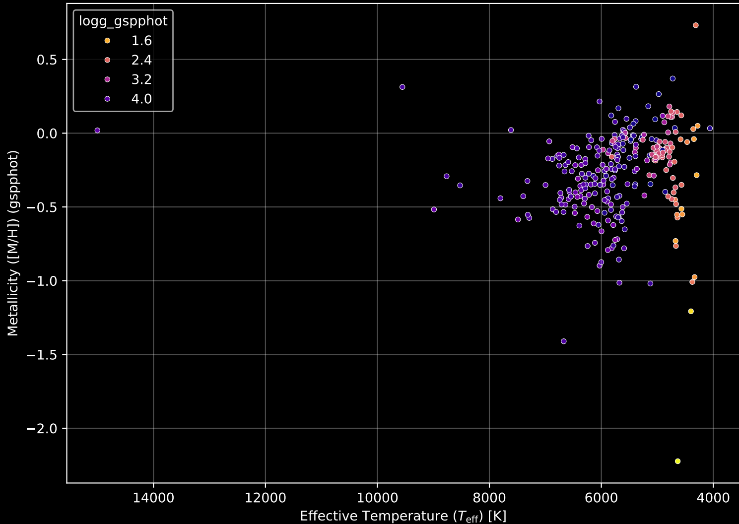
GALAH DR4 Field: [7191] Stellar Population Parameters (n= 270)
